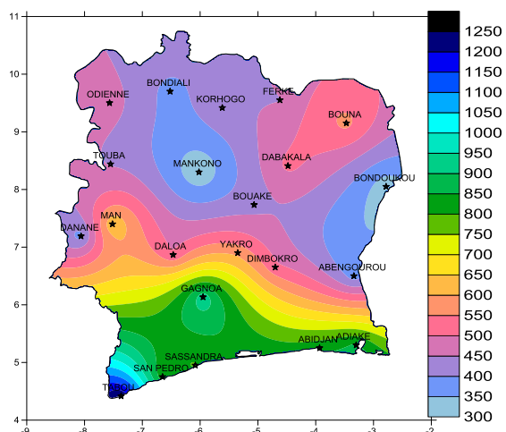
Fig 3: Cumul pluviométrique (mm) du 1 janvier au 10 Juillet 2016
