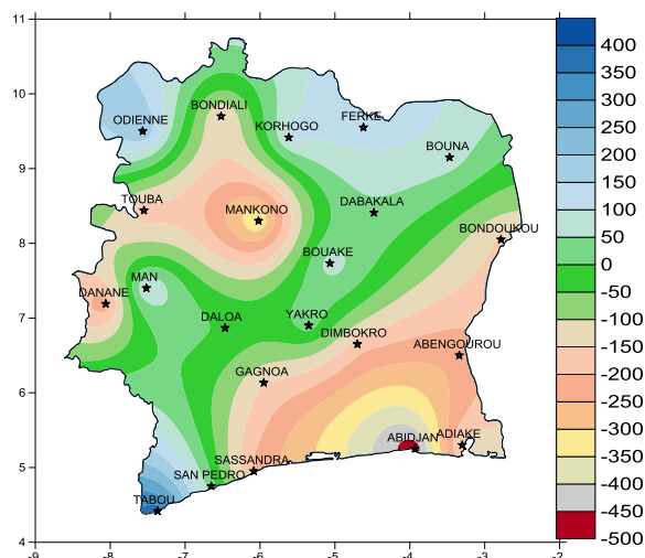
Fig 4 : Ecart entre Cumuls pluviométriques du 1 janvier au 10 Juillet 2016 et du 1 janvier au 10 juillet 2015
