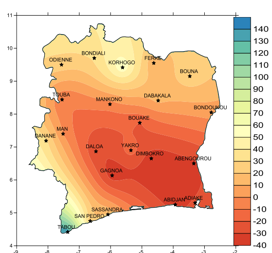
Fig. 9: Bilan hydrique climatique (mm) du 1 au 10 Juillet 2016
