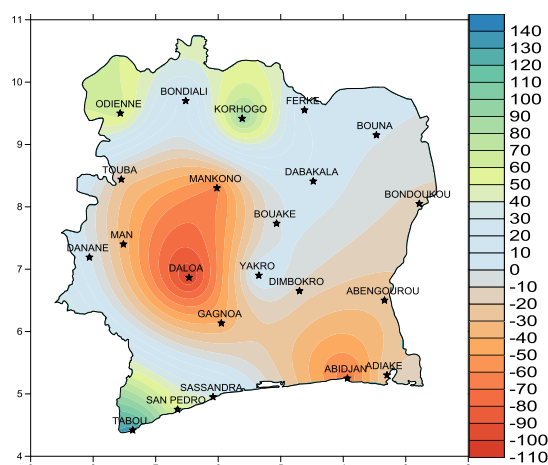
Fig2 : Ecart entre la pluviométrie (mm) du 1 au 10 Juillet 2016 et du 1 au 10 Juillet 2015
