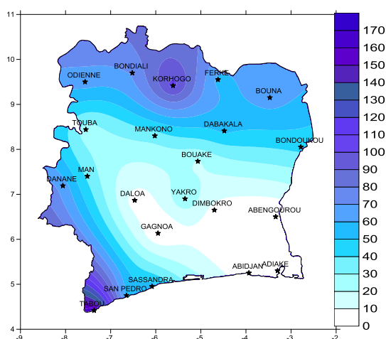
Fig1: Pluviométrie totale (mm) du 1 au 10 Juillet 2016
