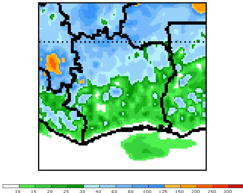
Figure 10 : prévision de la pluviométrie du 14 au 21 Juillet 2016 (source : NOAA, climate Prédiction Center)
